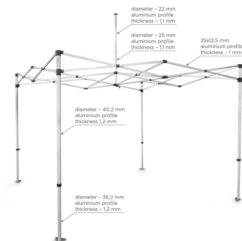
Hliníkové profily: nohy 40,2 / 36,2 mm, ramená 25 x 12,5 mm, stožiar 25 / 22 mm
