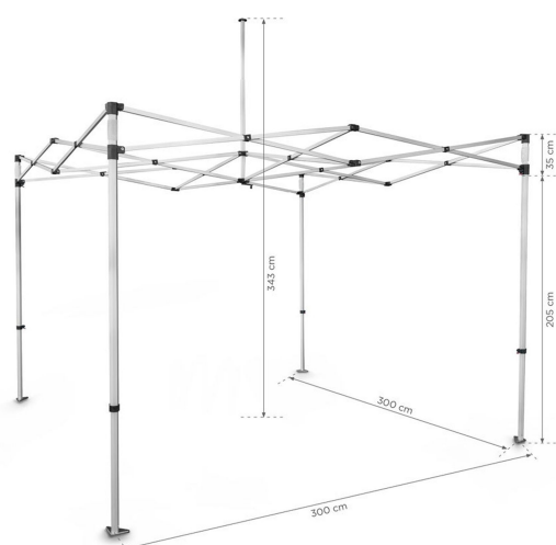
Rozmery konštrukcie: 300 x 300 cm, podchodná výška 205 cm, celková výška 343 cm
